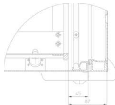
Schwingraum vermaßt
