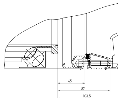
Schwingraum vermaßt
