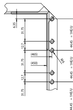
Lochbild vermaßt
