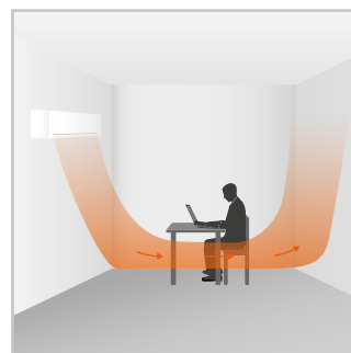
Zugluftfreie Luftführung im Heizbetrieb
