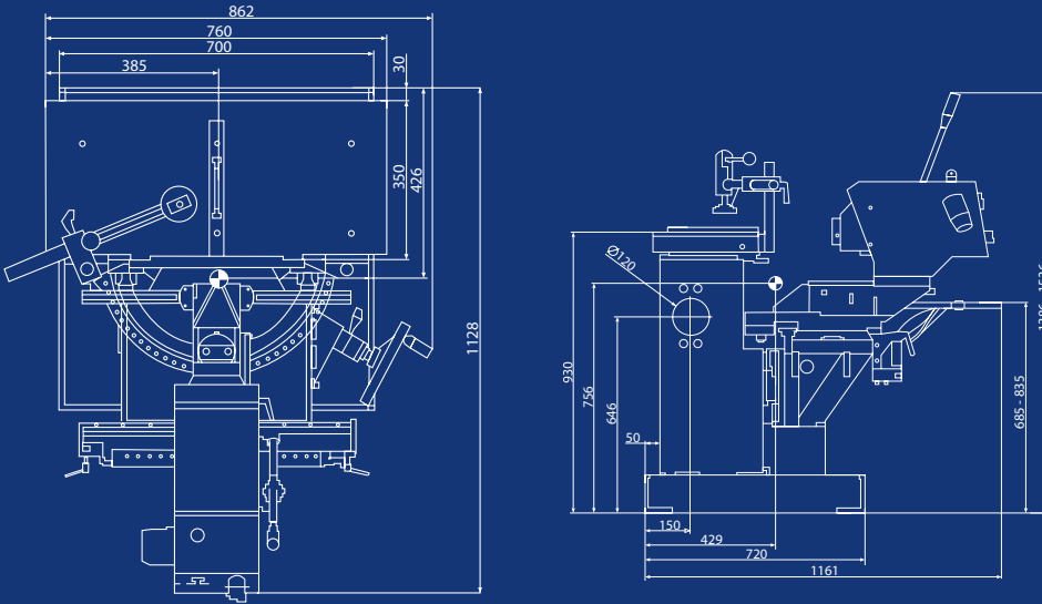
LB 780 schwenkbar
