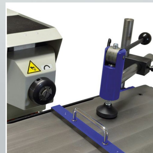
Drehzahl 1.500 und 3.000 UpM mit Bremseinrichtung
