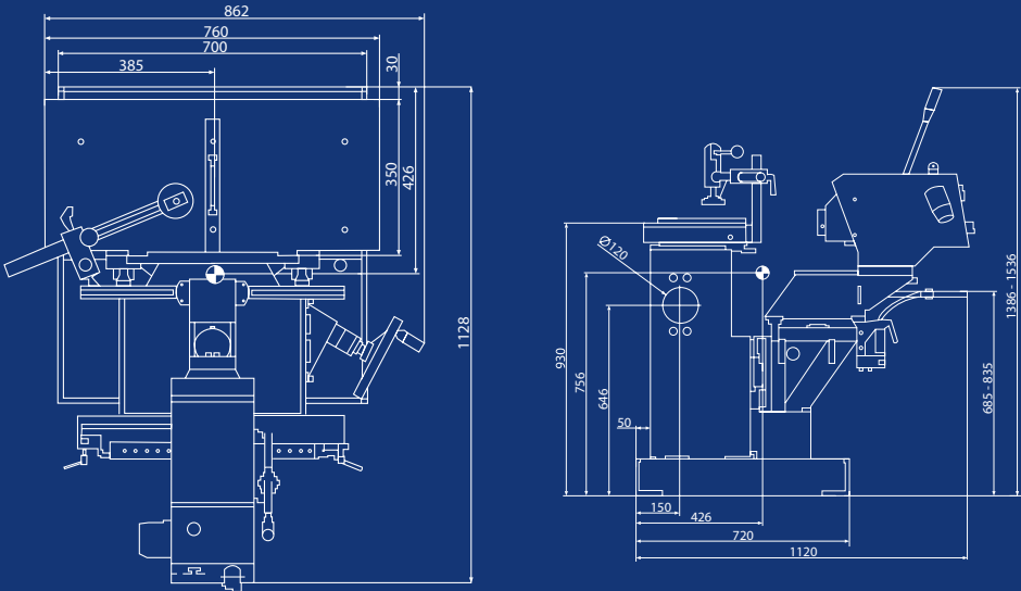
LB 780
