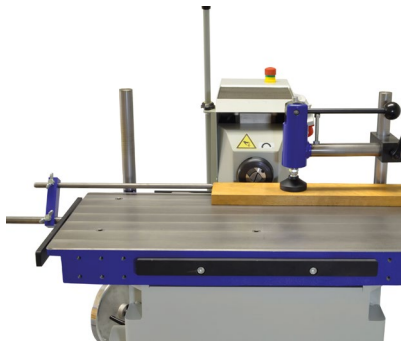
Verstellbarer Seitenanschlag
