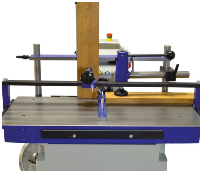
Spannbrücke zum senkrechten Spannen von Werkstücken
