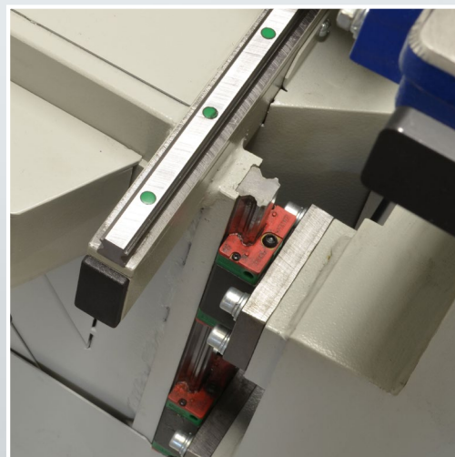
Verstellachsen in leichtlaufenden Profilführungen
