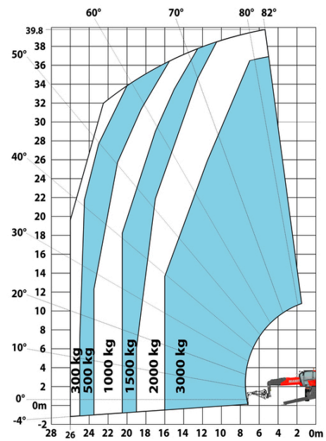
Maschine auf abgesenkten Stabilisatoren mit 3000 kg Windengalgen (Metric)
