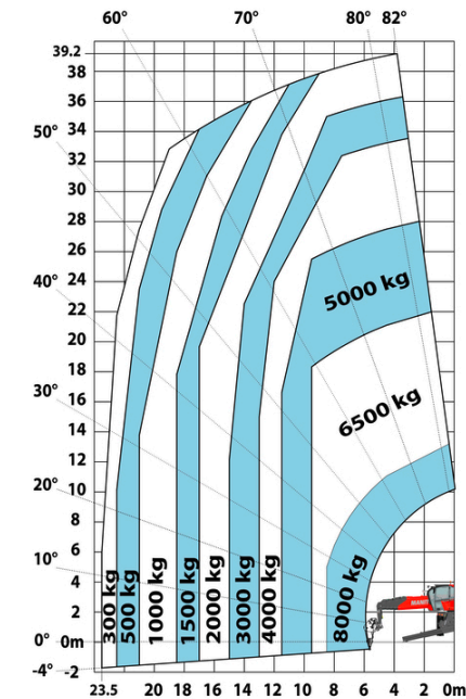
Maschine auf abgesenkten Stabilisatoren mit Winde 8000 kg (Metrisch) Drehung mit abgelassenen Stützen und 2 to jib (Metrisch)
