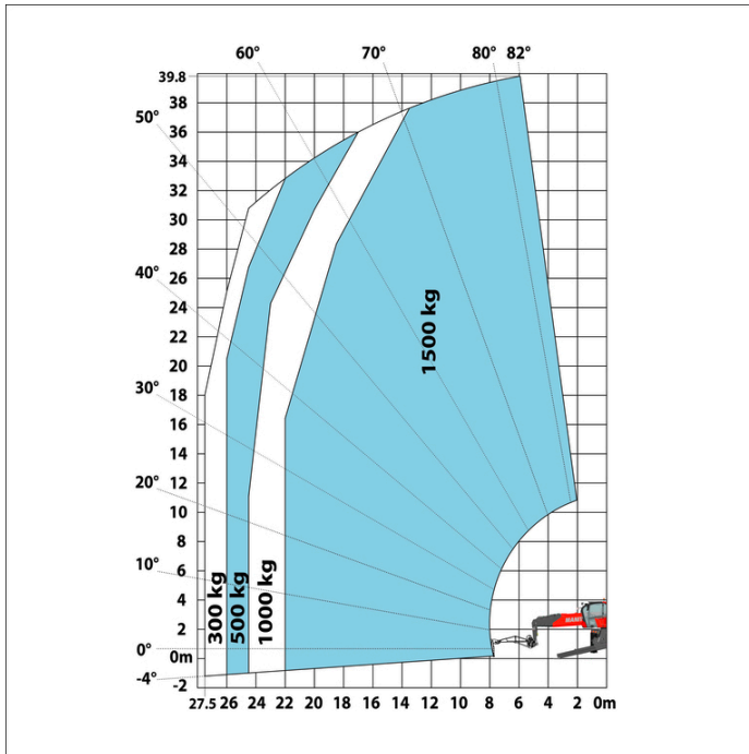
Maschine auf abgesenkten Stabilisatoren mit 1500 kg Winde (Metrisch)
