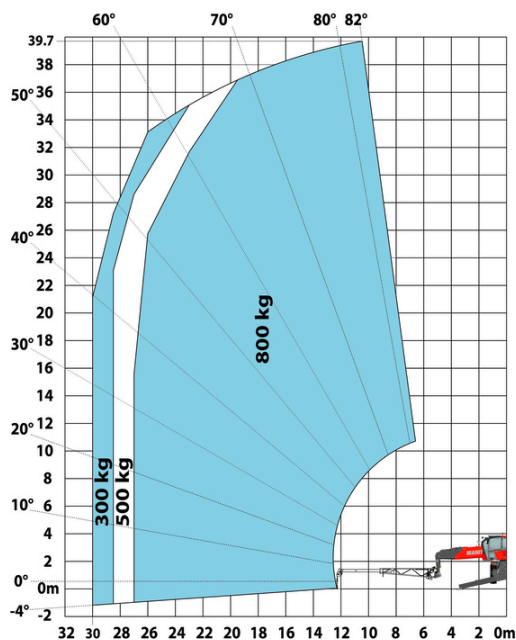
Maschine auf abgesenkten Stabilisatoren mit ausfahrbarem Windenarm (Metrisch)
