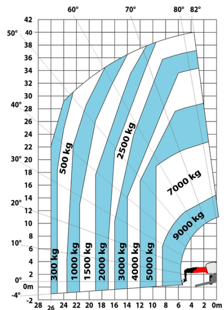
Maschine an abgesenkten Stabilisatoren mit Haken 9000 kg (Metrisch)
