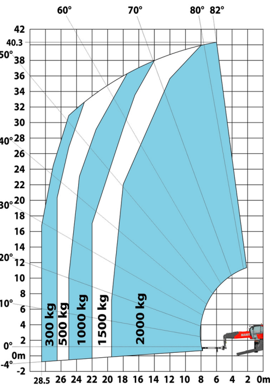
Maschine auf abgesenkten Stabilisatoren mit Winde 8000 kg (Metrisch) Drehung mit abgelassenen Stützen und 2 to jib (Metrisch)
